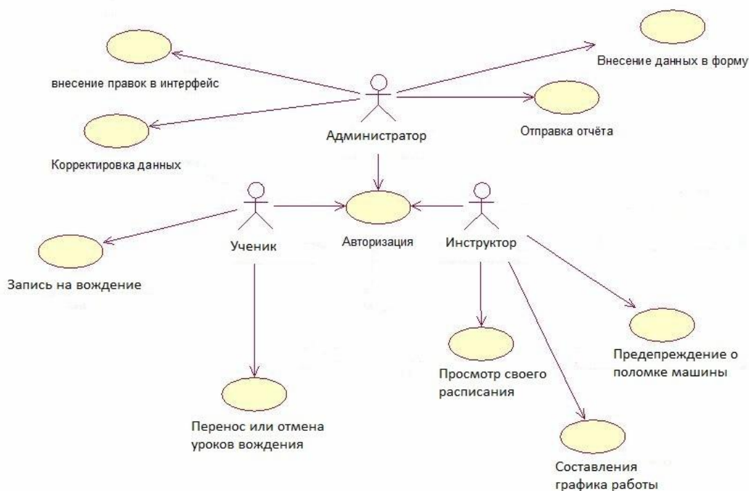
Рисунок 1 - Информационная модель
