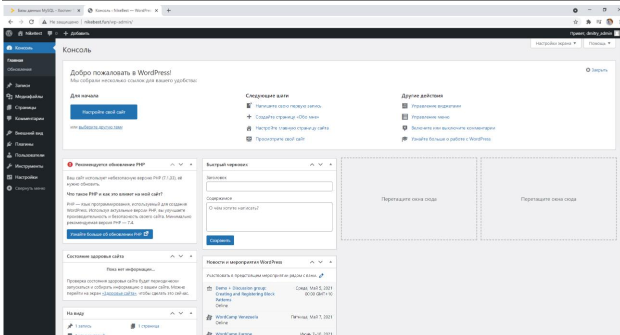
Рис. 10 Админпанель WordPress
