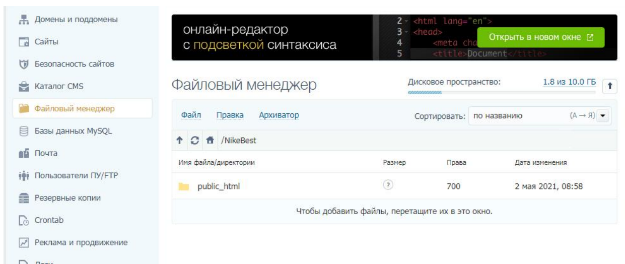
Рис. 5 Файловый менеджер
