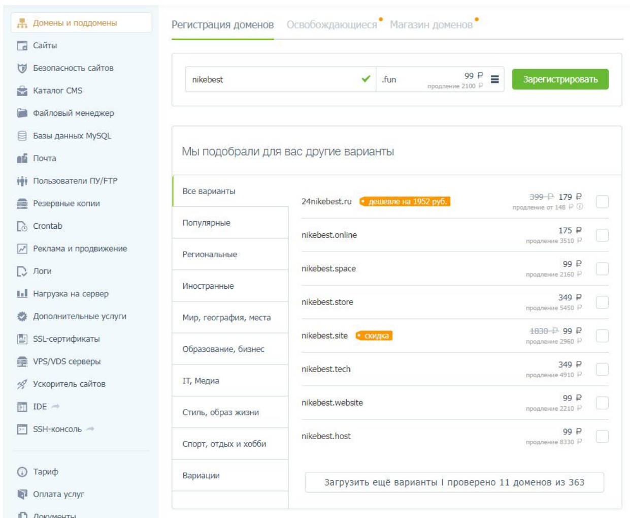
Рис. 3 Регистрация домена
