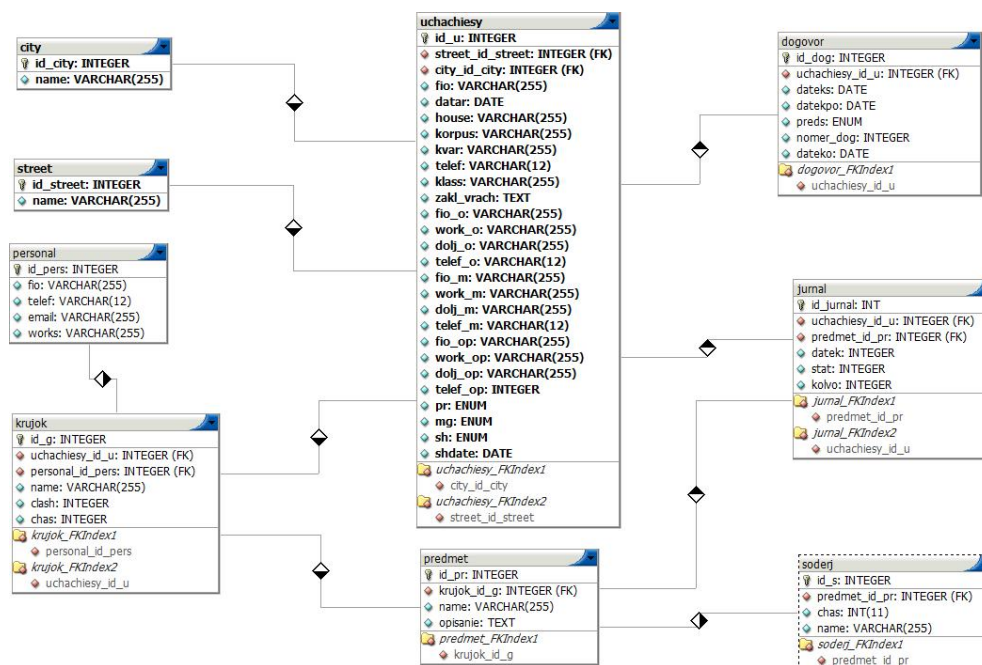
Рисунок 1 – Физическая модель БД
