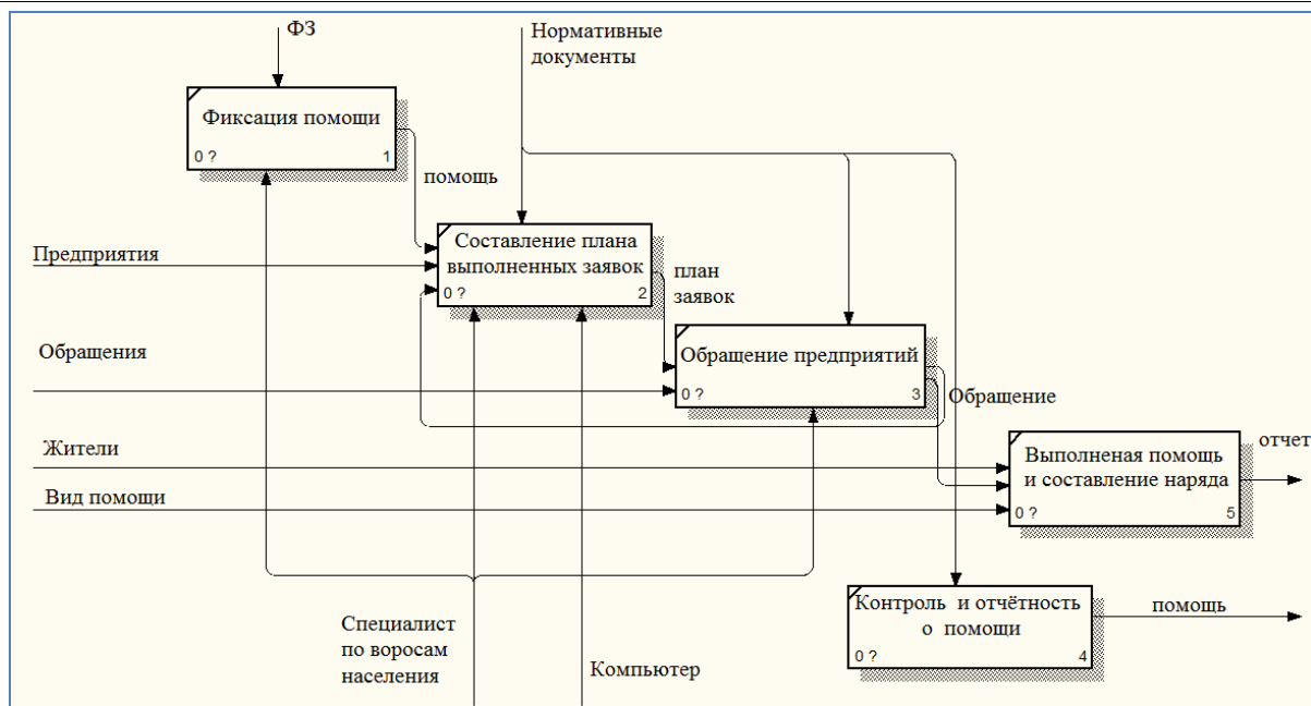
Рисунок 2—Главная диаграмма бизнес-процесса
