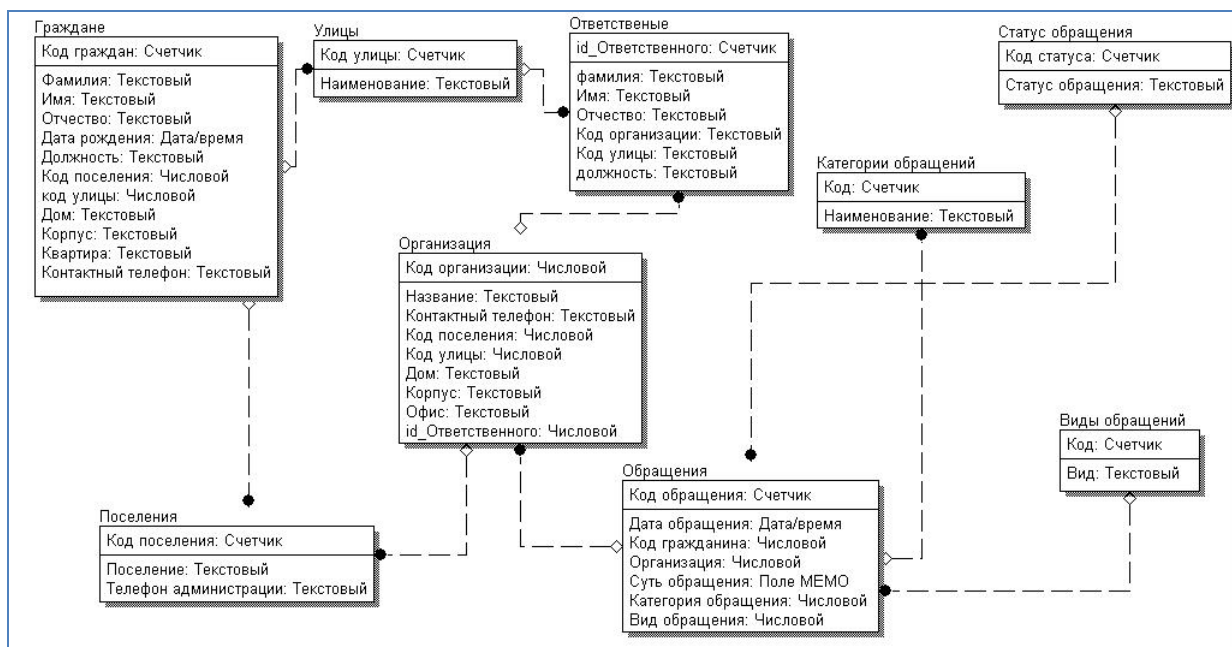
Рисунок 3 – Физическая модель БД
