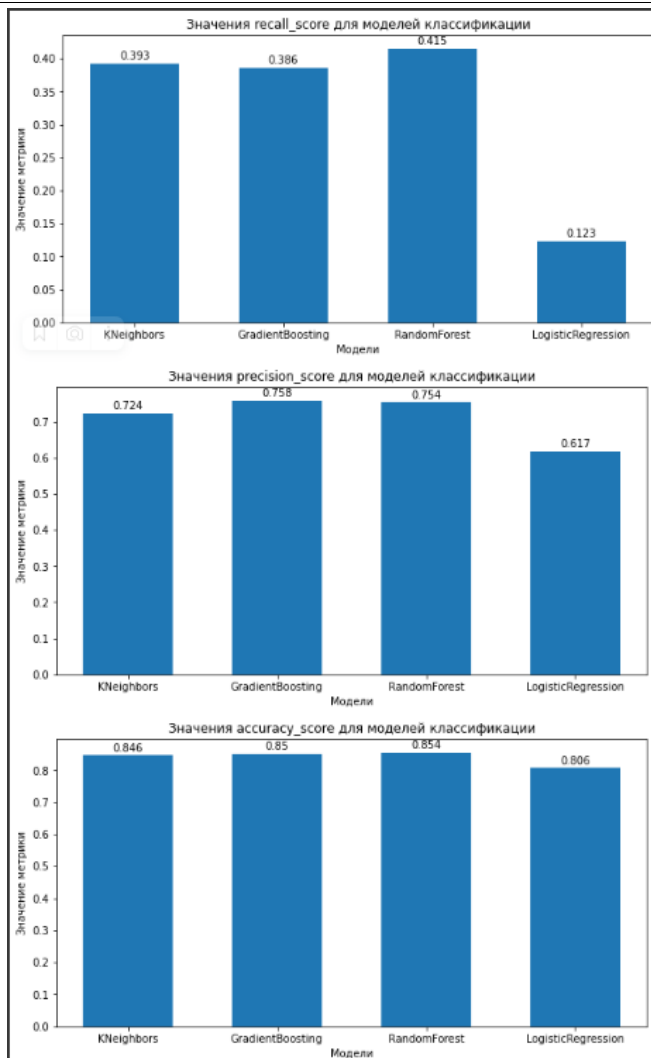
Рисунок 14 - Оценка метрик
